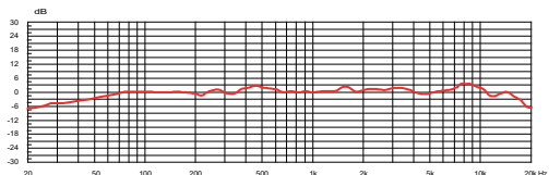
Частотная хар-ка
